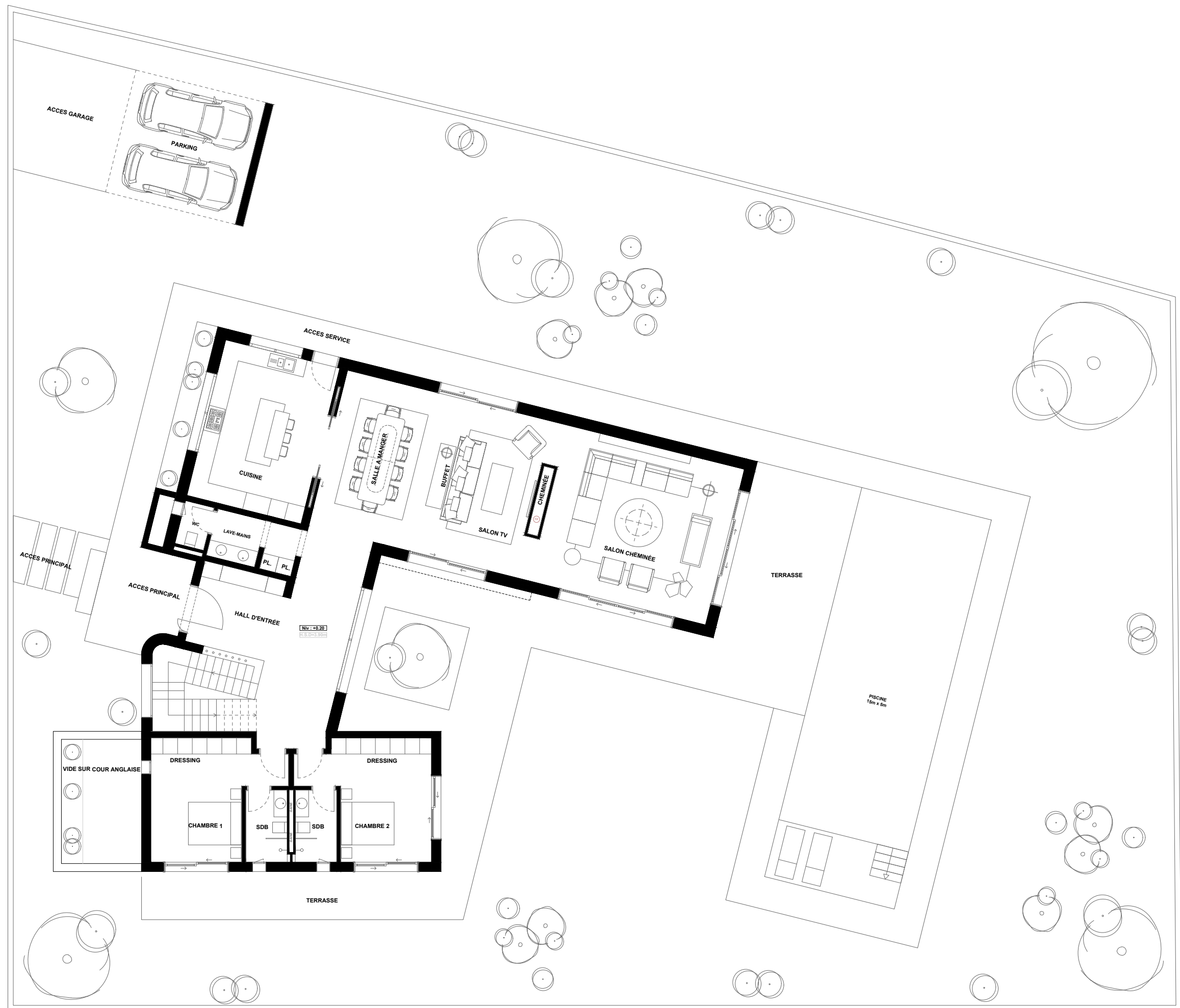
01 — PLAN RDC
