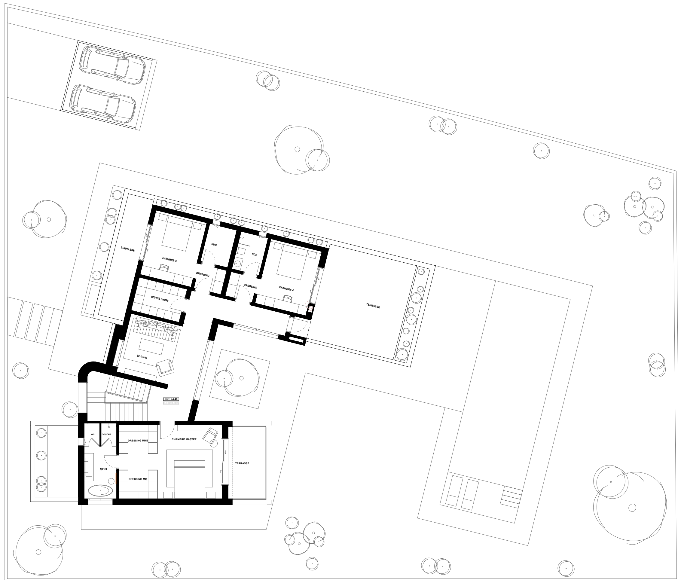
02 — PLAN ETAGE
