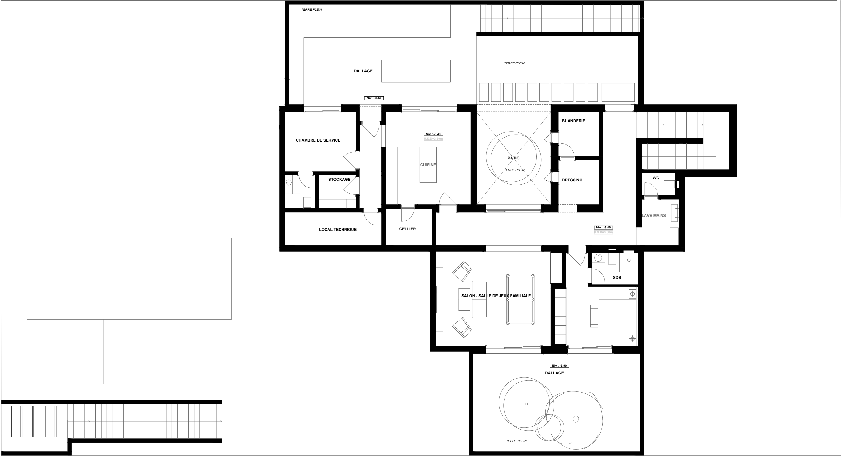
03 — PLAN SOUS SOL
