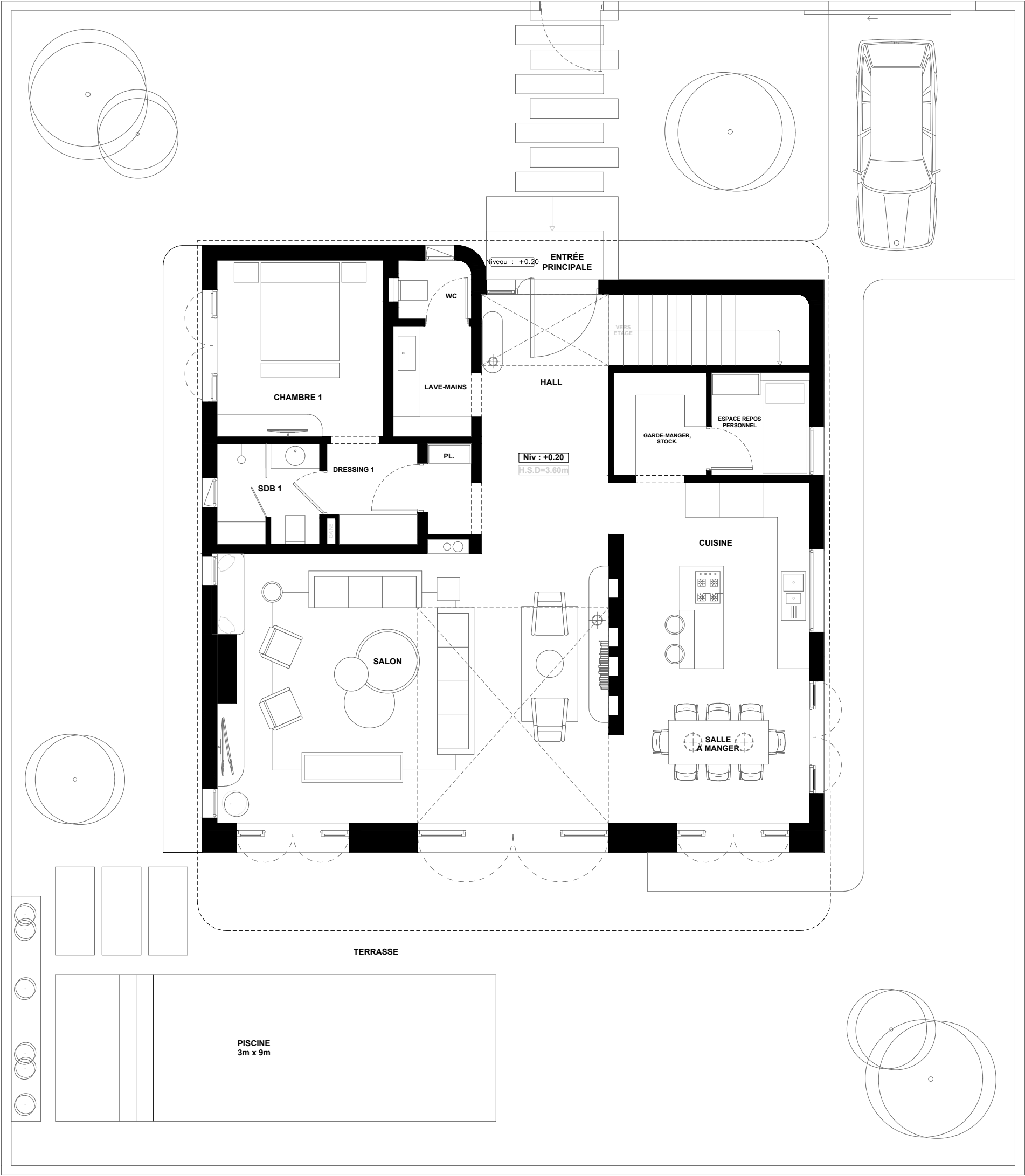
01 — PLAN RDC
