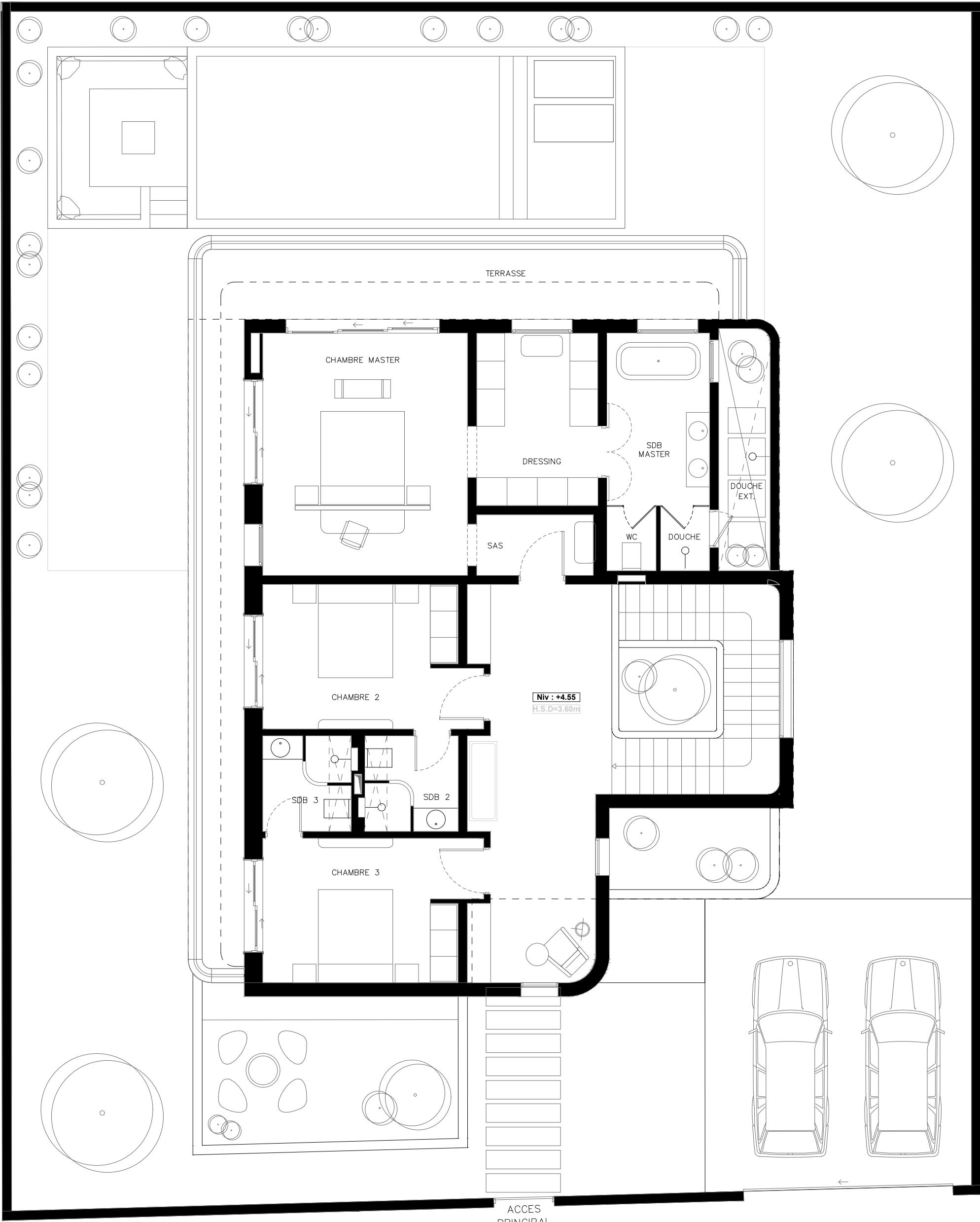
02 — PLAN ETAGE
