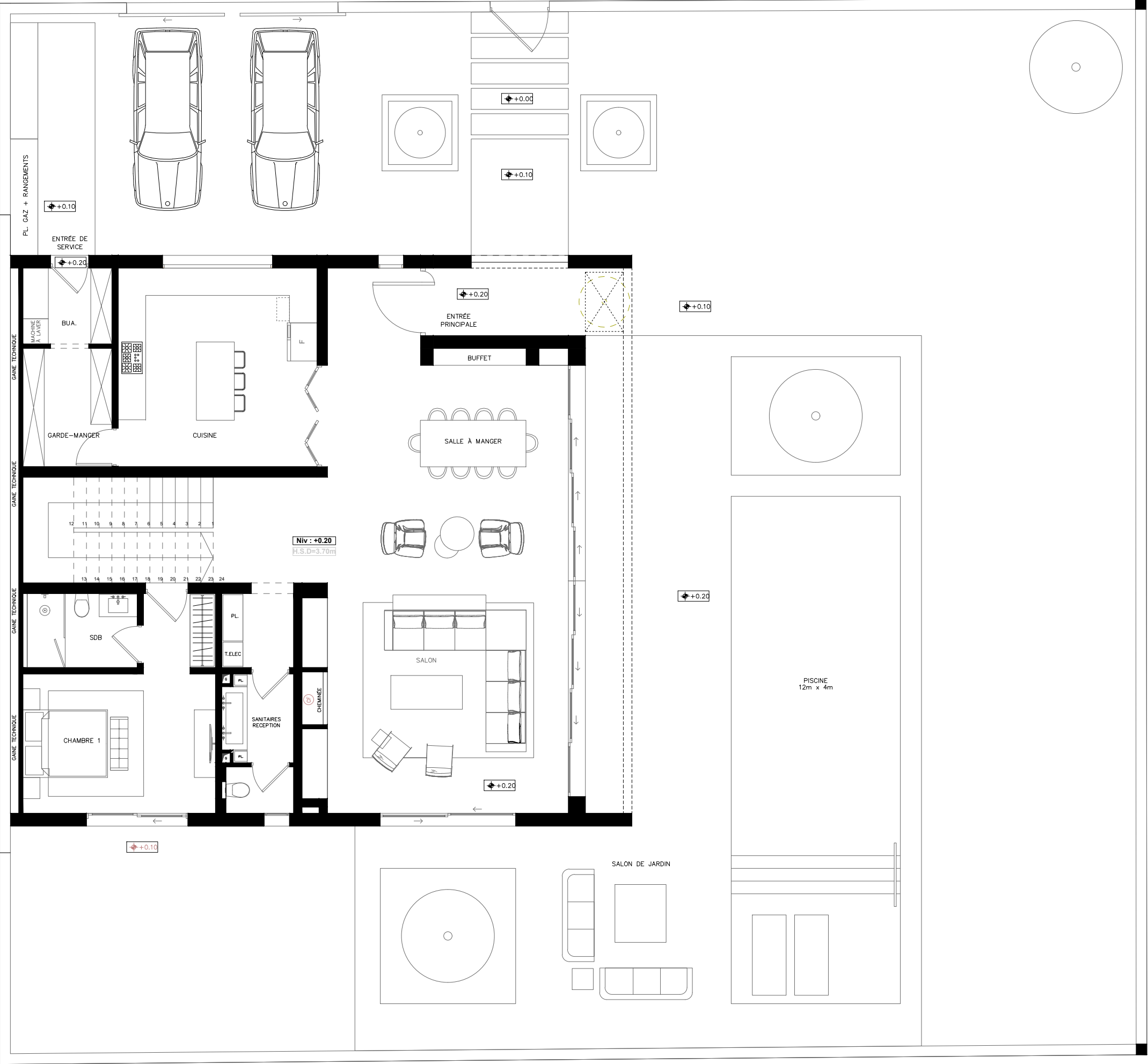
01 — PLAN RDC
